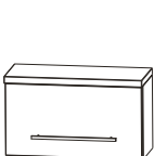
OBERSCHRANK » Maße (B/H/T): ca. 60 x 34 x 23 cm
