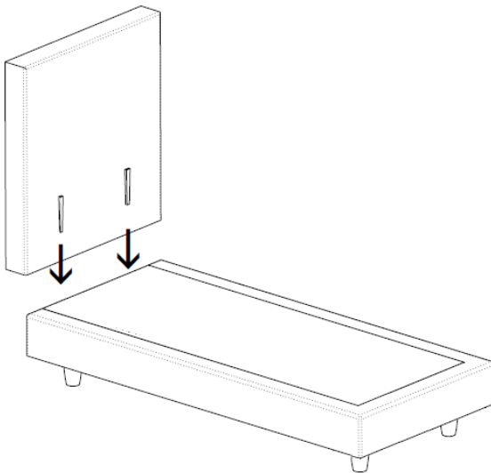
Abb. 5 Montage Kopfbrett
