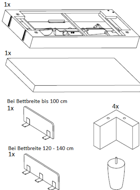
Abb. 16 Komponenten Einzelbett mit elektrischer Verstellung
