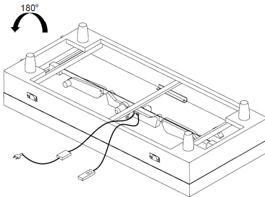
Abb. 30 Drehen der Box auf die Füße
