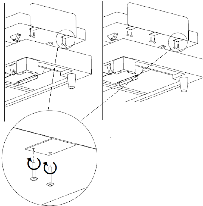
Abb. 53 Montieren des Matratzenhalters
