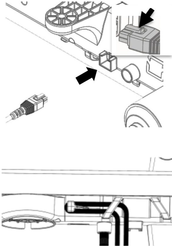
Abb. 49 Anschluss Fernbedienung
