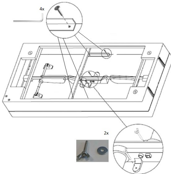
Abb. 19 Verschrauben der Motorbox
