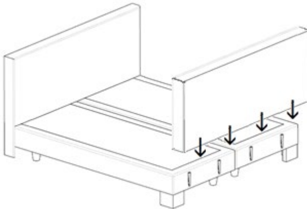
Abb. 14 Montage Fußbrett
