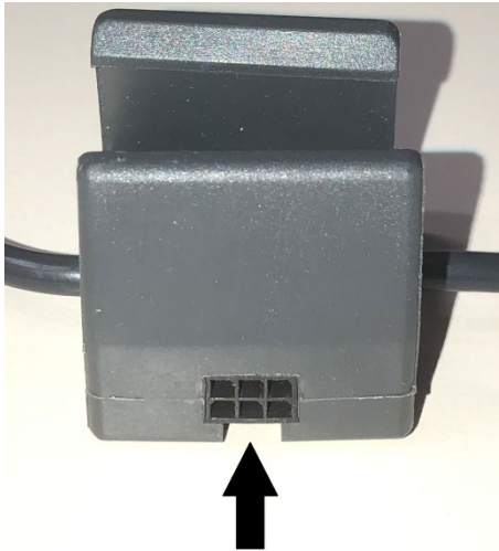
Abb. 60 Anschlussstück im Synchronkabel
