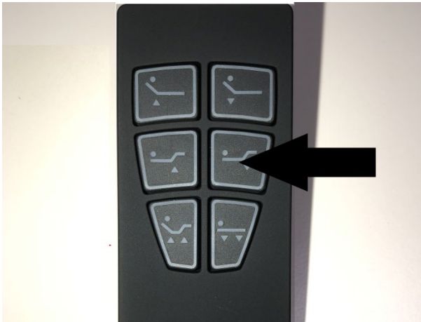
Abb. 54 Herunterfahren der Fußteile
