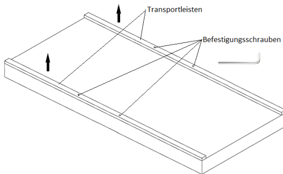
Abb. 17 Demontage der Transportleisten
