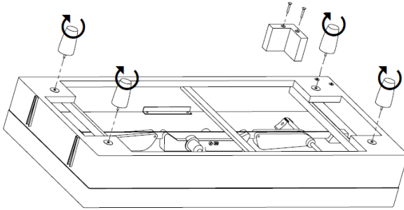
Abb. 20 Eindrehen bzw. Anschrauben der FüÙe
