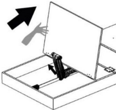
Abb. 67 Anheben Kopfteil für Notabsenkung
