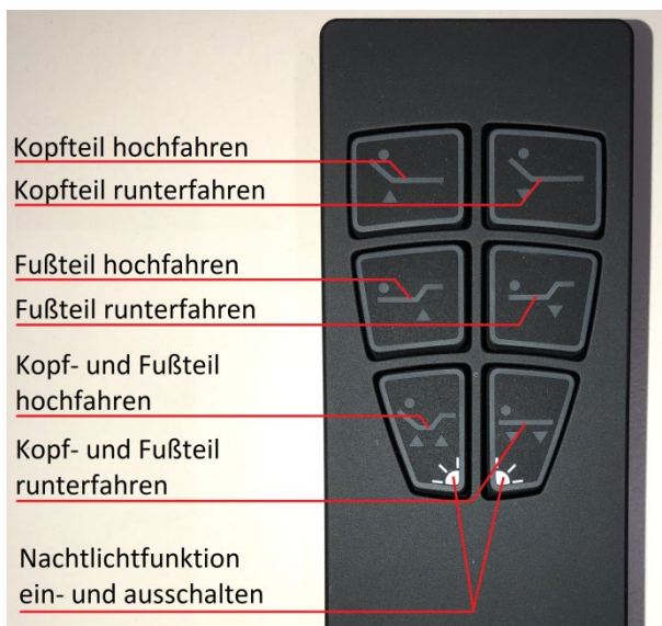
Abb. 63 Beschreibung Funkfernbedienung
