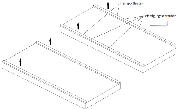
Abb. 37 Demontage der Transportleisten
