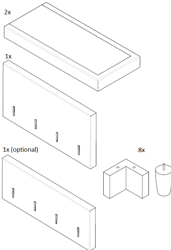
Abb. 8 Komponenten Doppelbett
