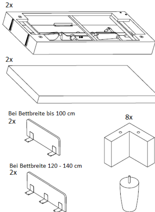
Abb. 36 Komponenten Doppelbett
