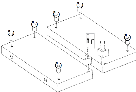
Abb. 10 Eindrehen bzw. Anschrauben der FüÙe
