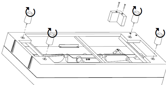
Abb. 40 Eindrehen bzw. Anschrauben der FüÙe
