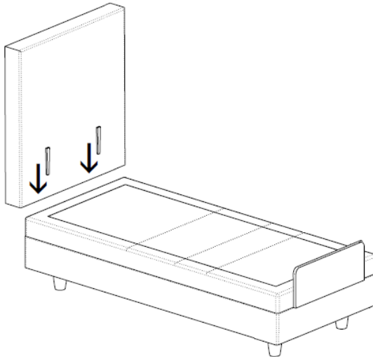
Abb. 34 Montage Kopfbrett
