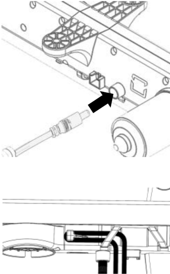
Abb. 48 Anschluss Netzadapter
