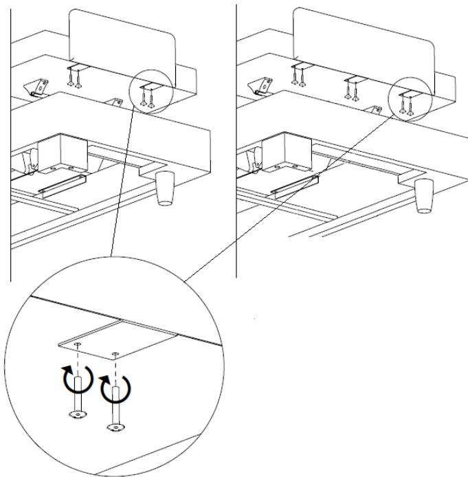
Abb. 32 Montieren des Matratzenhalters
