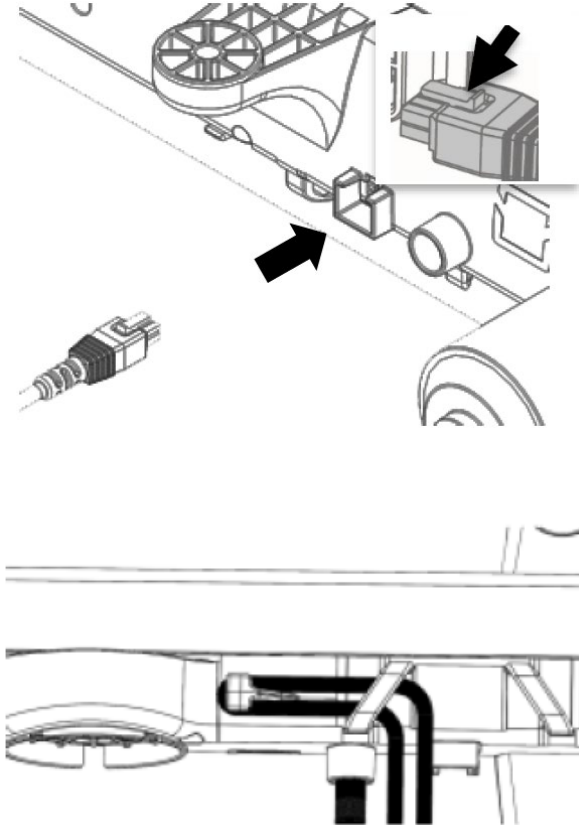
Abb. 29 Anschluss Fernbedienung
