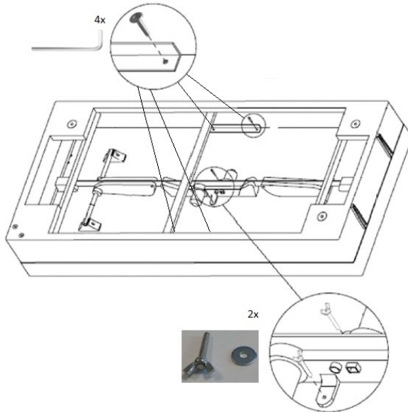
Abb. 39 Verschrauben der Motorbox
