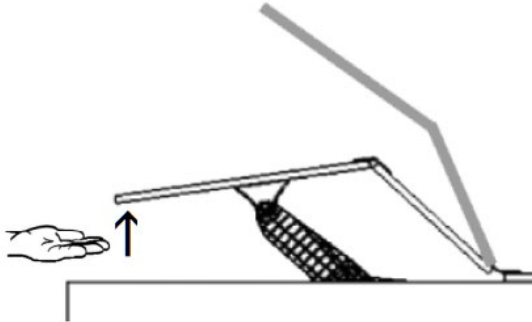
Abb. 69 Lösen der Verbindung zwischen Hebel und Fußteil
