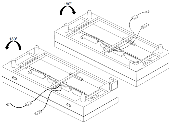
Abb. 50 Drehen der Boxen auf die Füße
