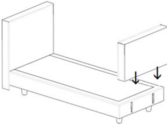
Abb. 6 Montage Fußbrett
