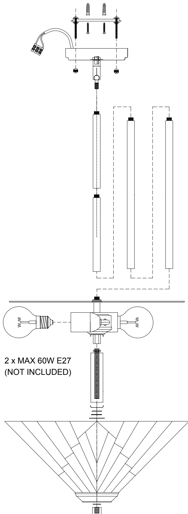
PENDANT MOUNTING
