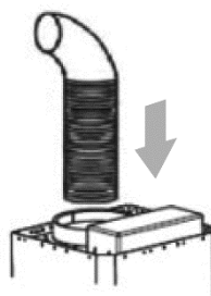
Kuva 2 Poistoilmaletkun asentaminen
