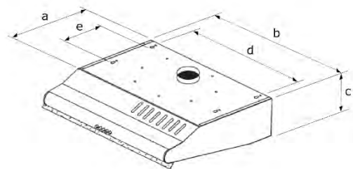
Fig. 9 Dimensões do aparelho
