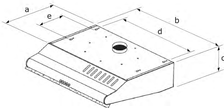
Abb. 1 Gerätemaße
