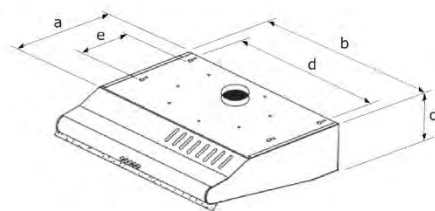
Kuva 1 Laitteen mitat
