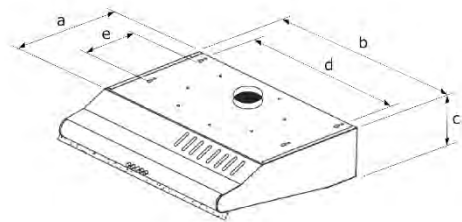
Bild 9 Apparatdimensioner
