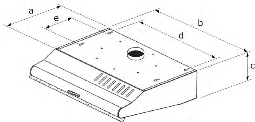
Fig. 1 Dimensiones del aparato
