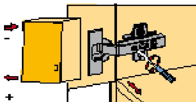
Auflagenverstellung
