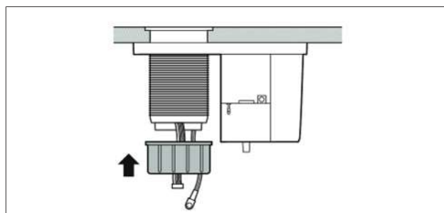
Abb. 8.16 Gerät befestigen
