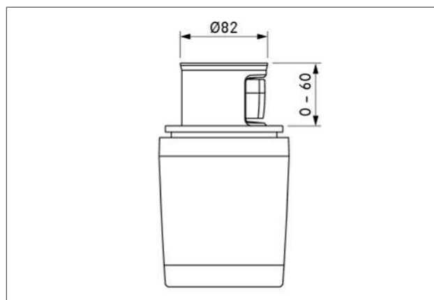
Abb. 3.3 Seitenansicht QVac
