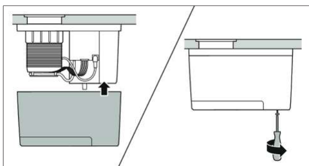
Abb. 8.19 Gehäuse aufschieben und festschrauben
