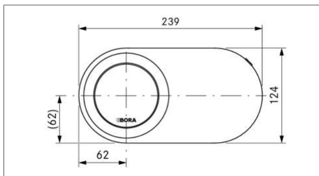
Abb. 3.2 Draufsicht QVac
