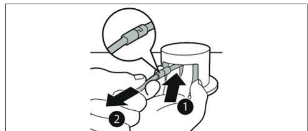
Abb. 6.2 Kupplung des Vakuumschlauchs herausziehen
