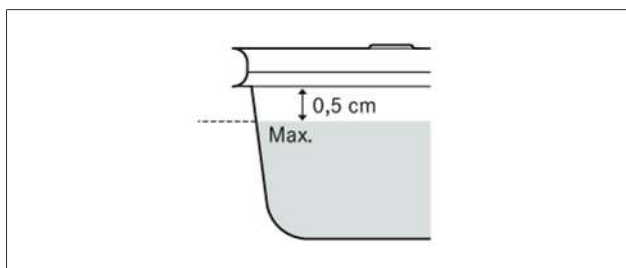
Abb. 5.4 Maximale Füllmenge
