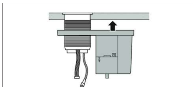
Abb. 8.15 Basiseinheit positionieren
