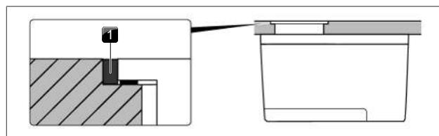
Abb. 8.21 Pop-up-Einheit verfugen
