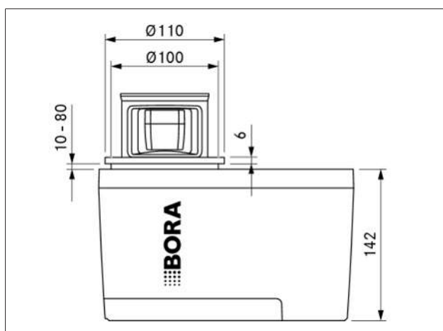
Abb. 3.1 Vorderansicht QVac
