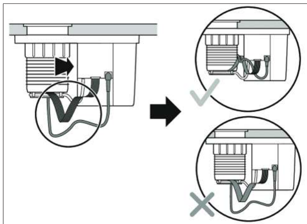
Abb. 8.18 Kabel anschließen
