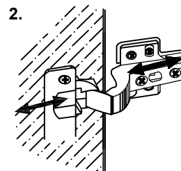
2. MOVE DOOR BACK OR
