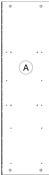
FI8997 1258x348x30mm
