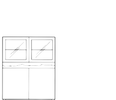
4 Türen, 1 Schubkasten, wahlweise mit LED-Glasbodenbeleuchtung B/H/T: ca. 122 x 148 x 40 cm
