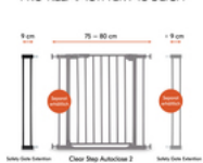
ZWEI VERLÄNGERUNGEN PRO KLEMMGITTER MÖGLICH
