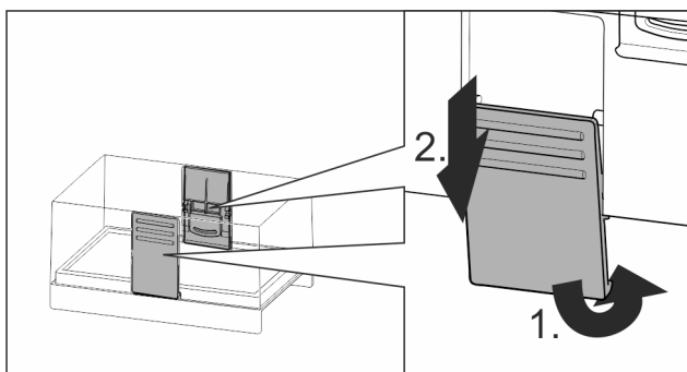
Fig. 168 Beispielhafte Darstellung des Eisfach-Trenners
