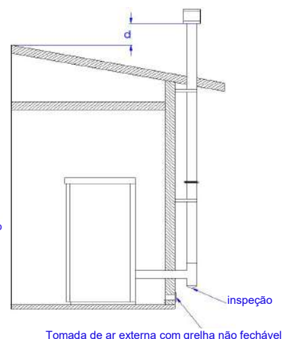
TUBO DE EVACUAÇÃO DE FUMOS EXTERNO
