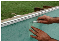
Fixing of the skimmer joint Fijación de la primera junta del skimmer Fixation du 1er joint de skimmer Befestigung der ersten Dichtung des Skimmers Fissaggio del primo giunto dello skimmer Bevestiging van de eerste pakking van de skimmer Fixação da primeira junta do skimmer
