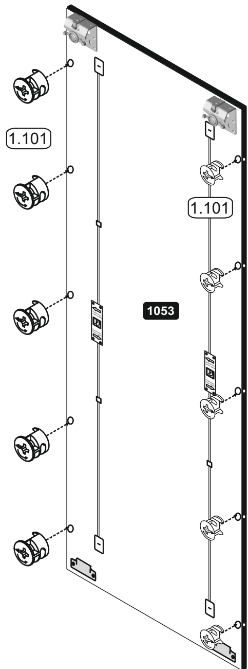
Korpus-Montage
