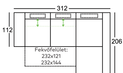
210-T-156-DL, 820-78 (220-T-156-DL, 810-78)
