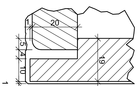
Detalj: Q (1:1)
