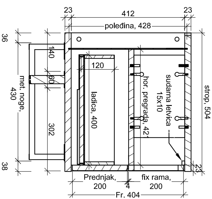
Presjek: V-V (1:8)
