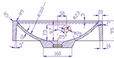
REZ A-A/ SECTION A-A
