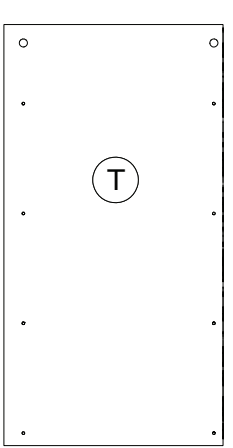
TR1957 778x405x18mm
