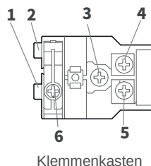
Klemmenkasten
