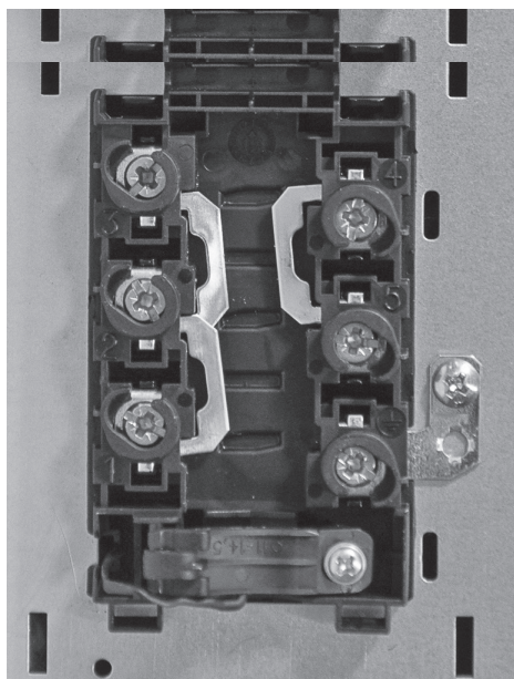
Anschlussbox geöffnet
