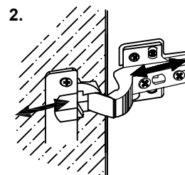
2. MOVE DOOR BACK OR FORWARD
