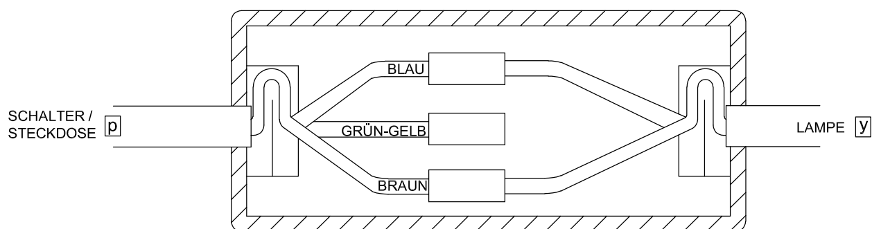
T16 ANSCHLUSSDOSE
