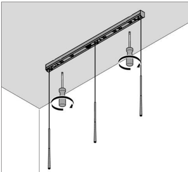
Abb. 5.5 Leuchte fixieren
