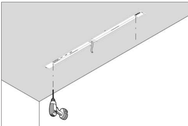
Abb. 5.1 Montage mit Bohrschablone
