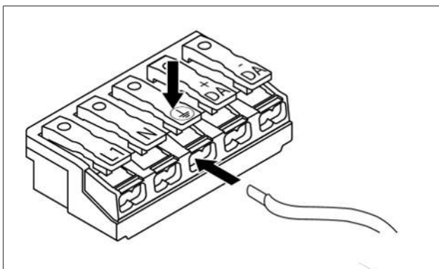
Abb. 5.6 Anschlussklemme
