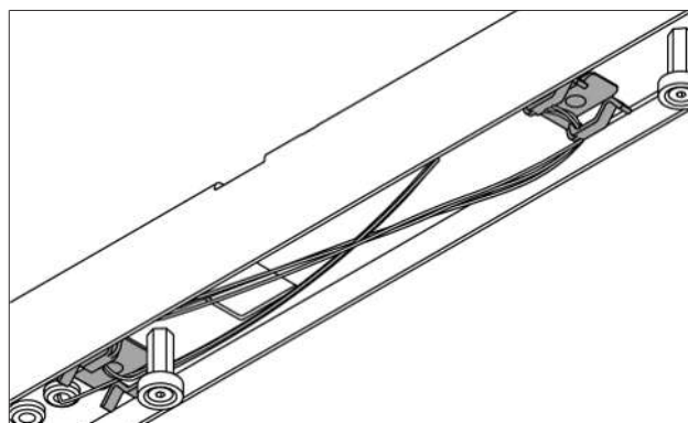
Abb. 5.9 Kabel verstauen
