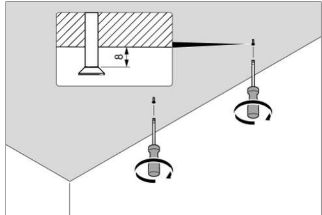
Abb. 5.2 Befestigungsmaterial vormontieren
