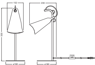
DECOR BELL TABLE PCR E27
