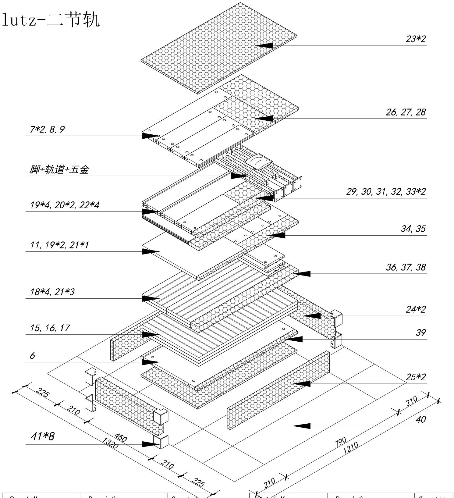
瓦尔特餐边柜拉槽利尼脚邮购包装图2-1
