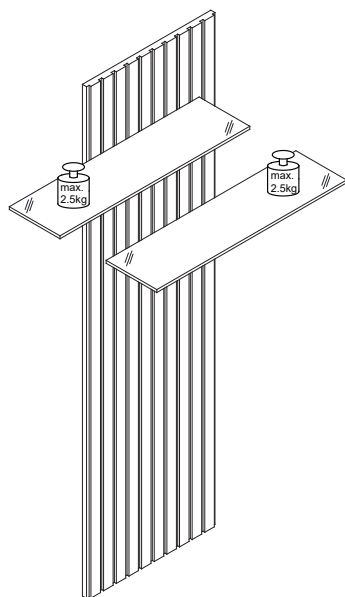
T08 - Aufsatzpaneel
