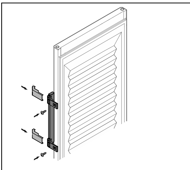
Fig. 27 Geschäumte Tür*
