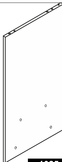
1025 736 x 394 mm
