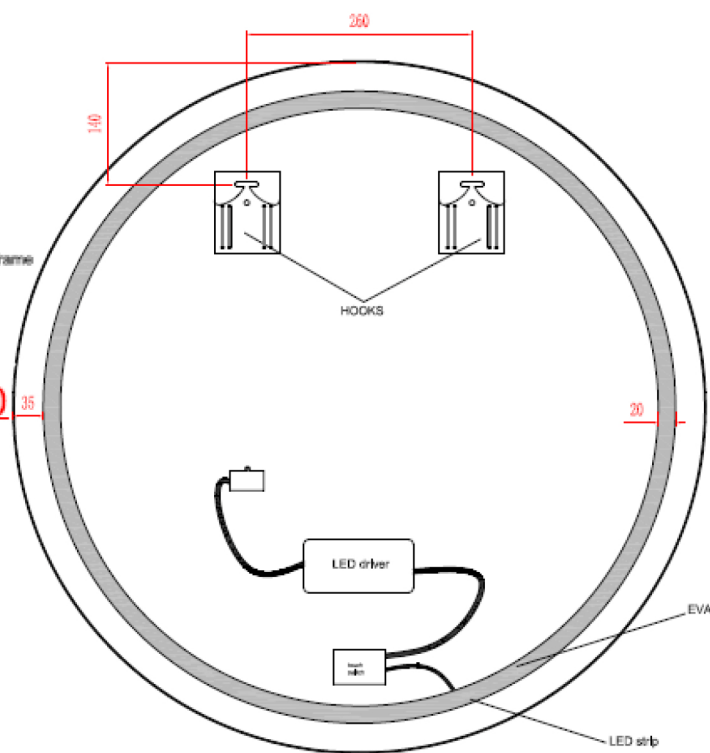
Rückseite/Backside
