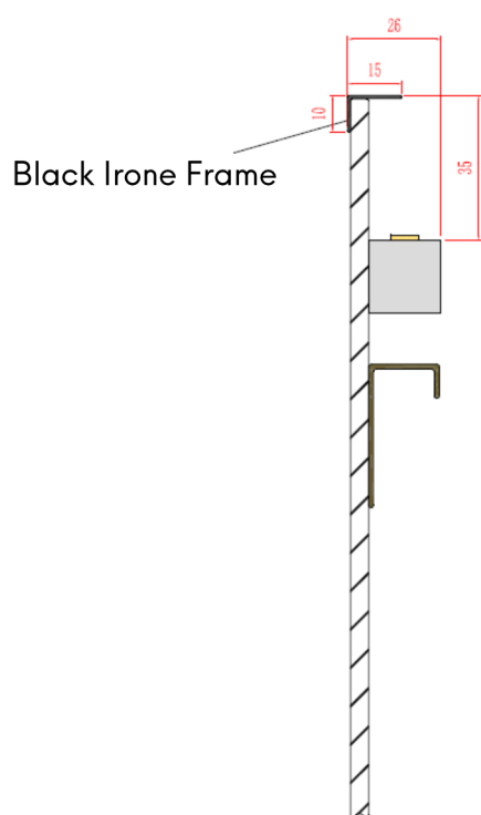
Seitenansicht/Sideview
