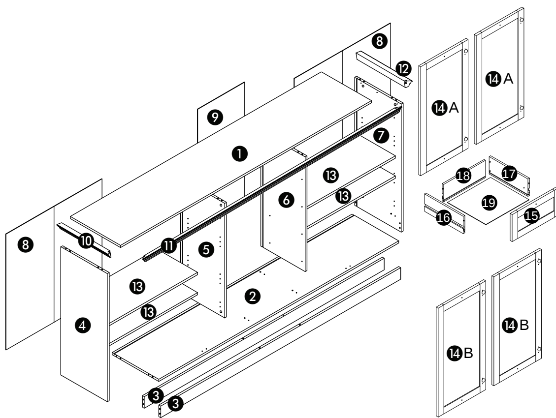
Dimensions / Abmessung in mm/
