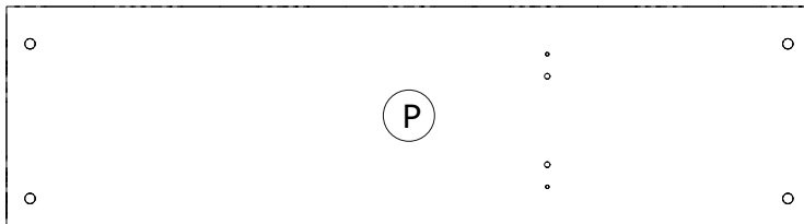
PI08030 1164x316x16mm
