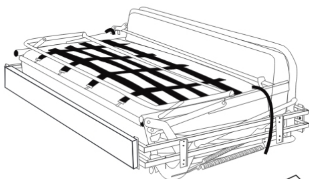
Mehanizam, sedeći deo
