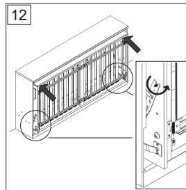
Rahmen oben einschwelen. Swivel the frame at the top.
