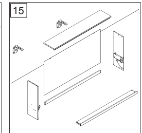
Korpus zerlegen. Disassemble corpus.
