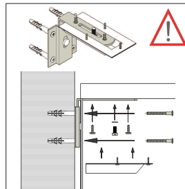
Befestigungswinkel unter dem Oberboden verschrauben. Screw the mounting bracket under the topsoil.
