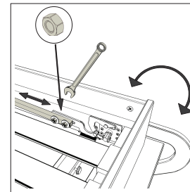
FußEinstellung. Foot adjustment.
