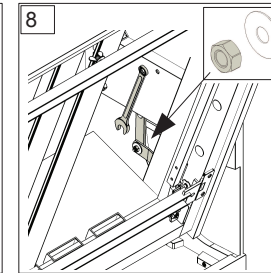
Mutter & Unterlegscheibe entfernen. Remove nut & washer .
