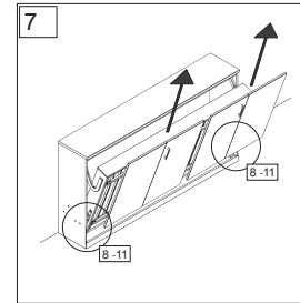
Frontteile herausnehmen. Lift out the front parts.
