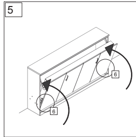
Bettrahmen hochklappen. Lift the bed frame.
