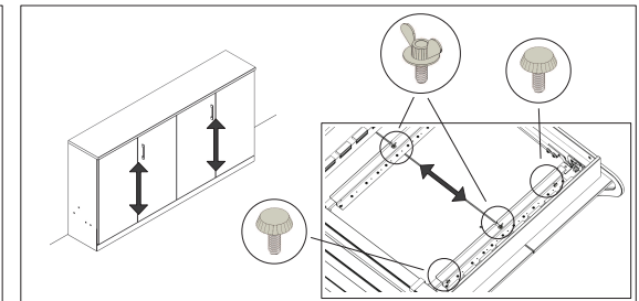
Höheneinstellung der Front über Rändelschrauben. Height adjustment of the front over knurled crews.
