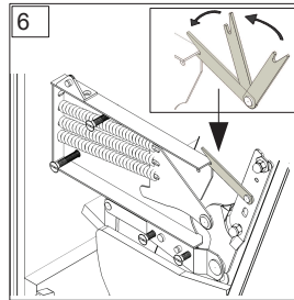
Die Montagehilfshaken arretieren. Lock the hook.
