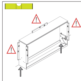
Seiten unterlegen, wenn uneben. Inferior sides, if uneven.
