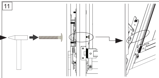
Untere Schraube durchdrücken. Press the bottom screw out of frame.
