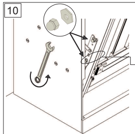
Hutmuttern & Exzenter entfernen. Remove cap nuts & eccentric.
