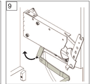
Verbindung trennen. Disconnect.
