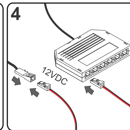
ZUBEHÖR BELEUCHUNG OŚWIETLENIE DODATKOWE P900ZBL1
