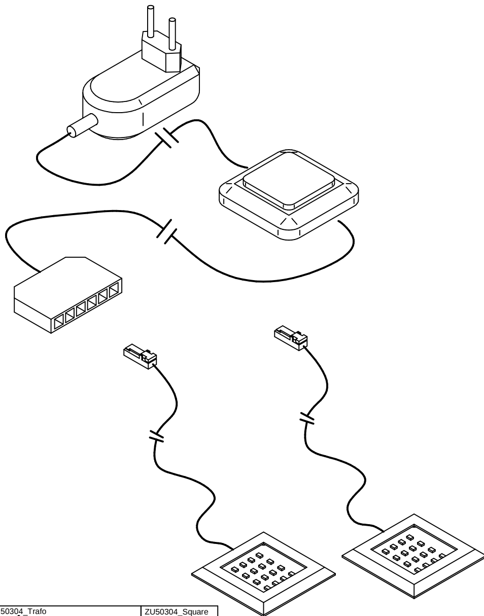
ZU50304_Trafo
