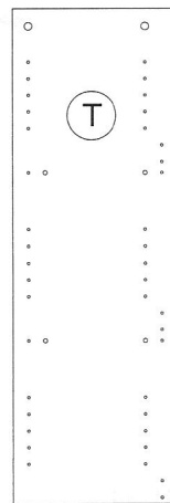
TR2184 952x321x18mm
