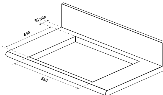
Für den flächenbündigen Einbau umlaufend min. 1,8 mm für die Silikonfuge berücksichtigen. Falzhöhe 7 mm
