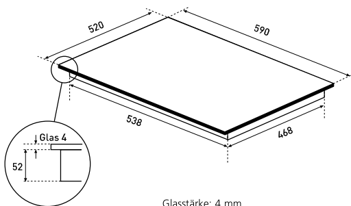
Glasstärke: 4 mm Eckradius: 8 mm
