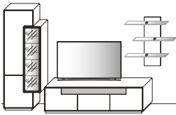
Kombination 0005 B/H/T: ca. 333 x 198 x 52 cm
