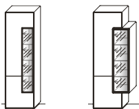
Zeilenschrank (Abb. 1) B/H/T: ca. 59 x 198 x 36 cm Zeilenschrank (Abb. 2) B/H/T: ca. 75 x 198 x 38 cm
