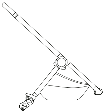
Gestell | frame
