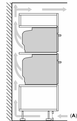
Einbau von zwei Geräten übereinander Luftaustausch
