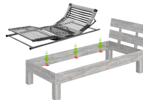
3-Punkt Auflage
