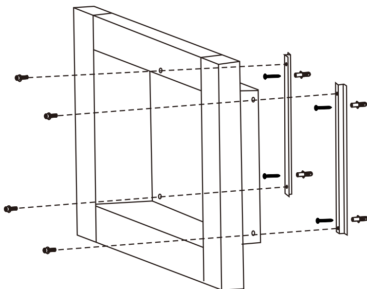
Montaje en pared (con soportes)
