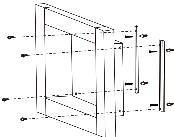
Montage mural (avec supports)
