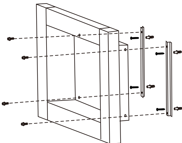
Montagem na parede (com suportes)
