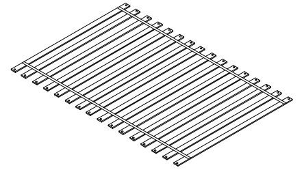
F-Slats (16pcs)
